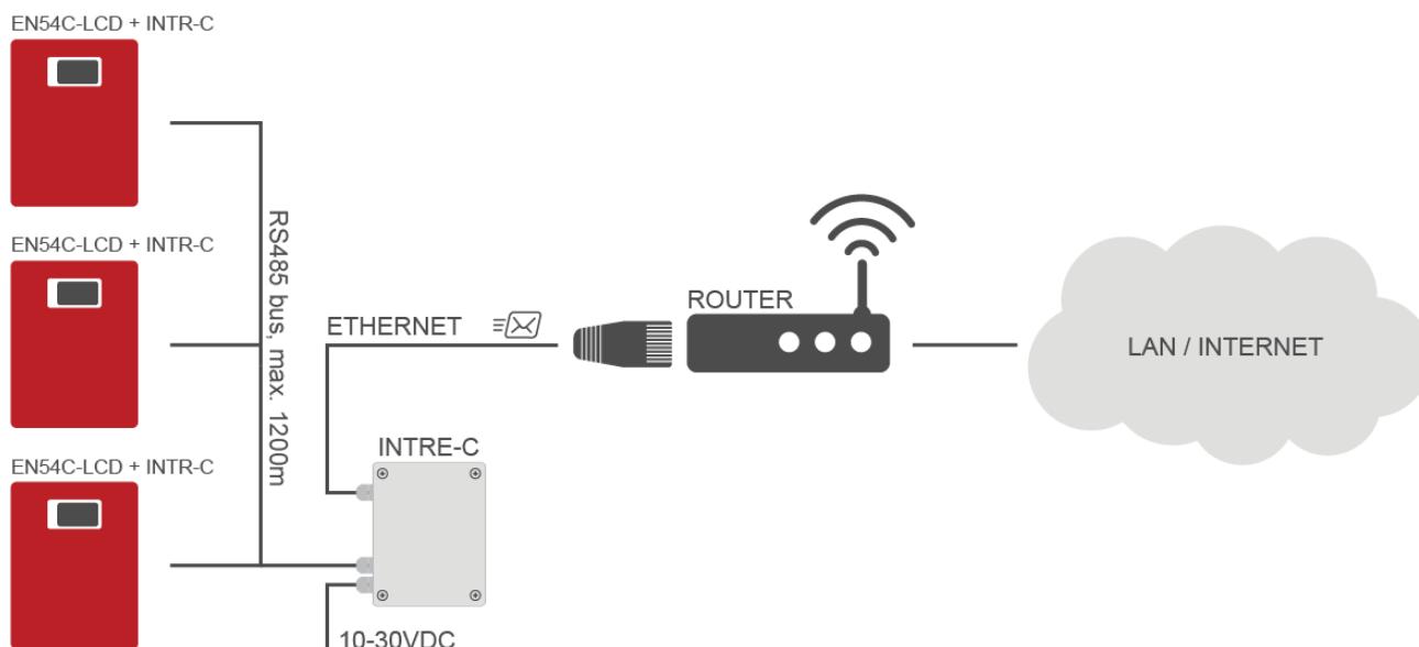
Rys. 1. Schemat poglądowy systemu zdalnego monitoringu zasilaczy.
